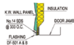
SECTION THRU' JAMB
