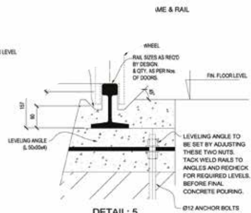
DETAIL: 5
