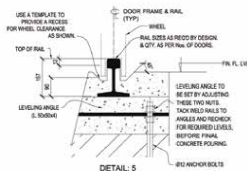
DETAIL: 5
