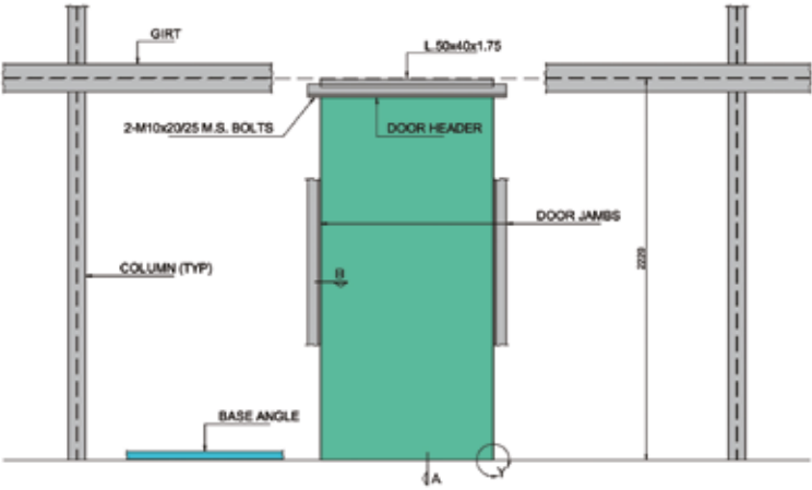
DOOR FRAME ERECTION
