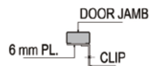
SECTION Y
