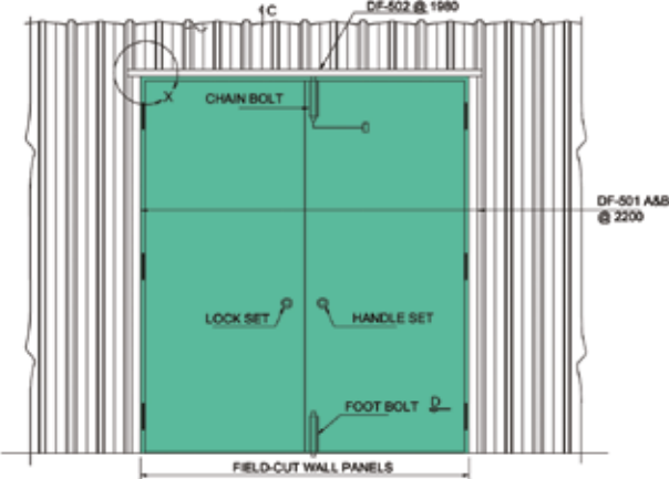
6'x7' WALK DOOR (1830X2134)
