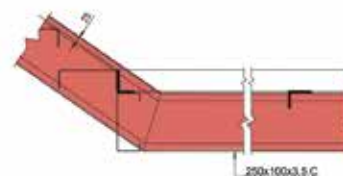
SECTION - E
